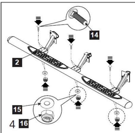
Abbildung 5 Schwellerrohre positionieren.
