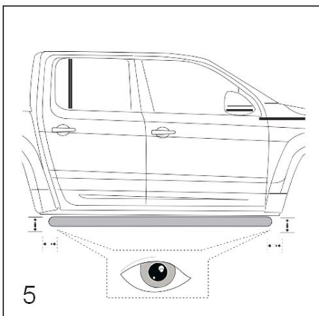
Figure 3 Identifier les supports (-3-, -4-, -5-, -6-, -7-, -8-) à l'aide des repères, et les fixer à la main, comme indiqué, avec les étriers de retenue (-9-, -10-, -11-), les vis -13- et les rondelles -12- sur le véhicule.
