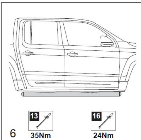
Figure 6 Visser les supports (-3-, -4-, -5-, -6-, -7-, -8-) sur le cadre, les fixer avec les vis -13- et les rondelles -12-. Couple de serrage : 35Nm Visser ensuite les tubes de seuil -1- et -2- avec les vis -14-, les rondelles -15- et les écrous -16- sur les supports. Couple de serrage : 24Nm Contrôler si tous les supports sont à la même distance du véhicule.
