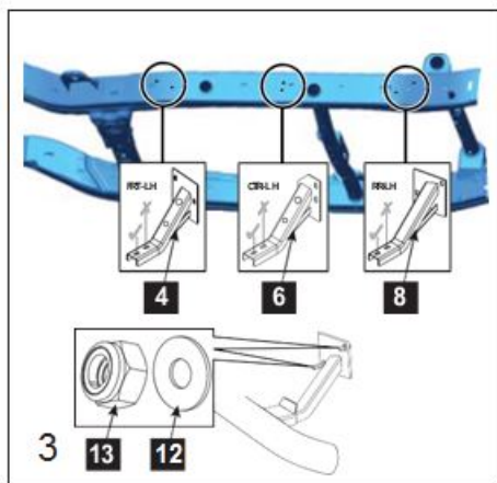
Abbildung 3 Identifizieren Sie die Halter (-3-, -4-, -5-, -6-, -7-, -8-) anhand ihrer Markierungen und befestigen Sie diese, wie dargestellt, mit den Haltebügeln (-9-, -10-, -11-), Schrauben -13- und Unterlegscheiben -12- handfest am Fahrzeug.
